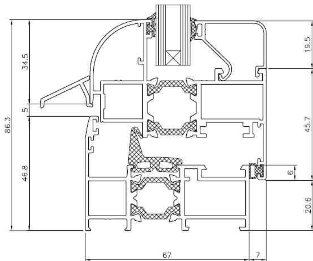
NUDO INFERIOR VENTANA MARCO 9801410 Y HOJA 9801420
