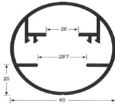
PASAMANOS REDONDO B-36
