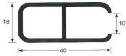
HOJA ACRISTALAMIENTO BARANDILLA B-23
