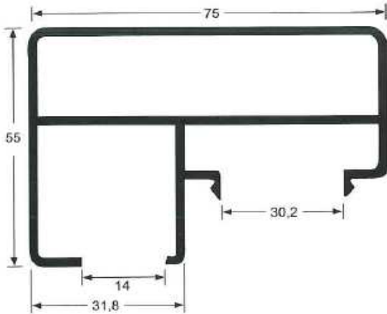
B-22 ANCLAJE BARANDILLA ACRISTALAR
