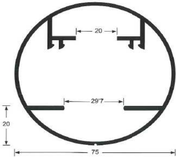
B-35 PASAMANOS REDONDO
