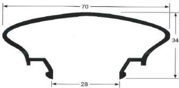
B-1 PASAMANOS BARANDILLA
