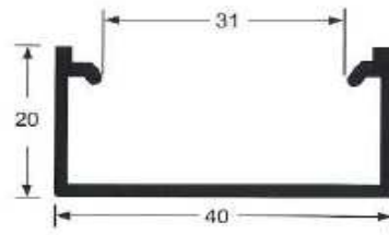
B-2 U TAPACANAL BARANDILLA
