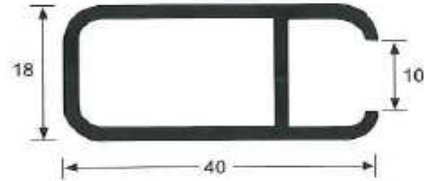
HOJA ACRISTALAMIENTO BARANDILLA B-21
