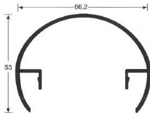
PASAMANOS REDONDO B-108
