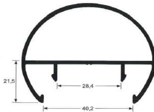
B-10 PASAMANOS REDONDO BARANDILLA
