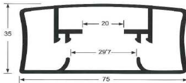
B-31 BARROTE DECORATIVO
